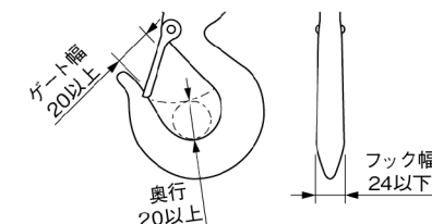
吊上げ式 適用フック寸法
