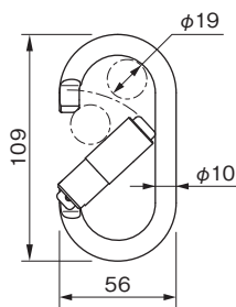
鉄 O型 アルミ環 ステン O型 アルミ環
